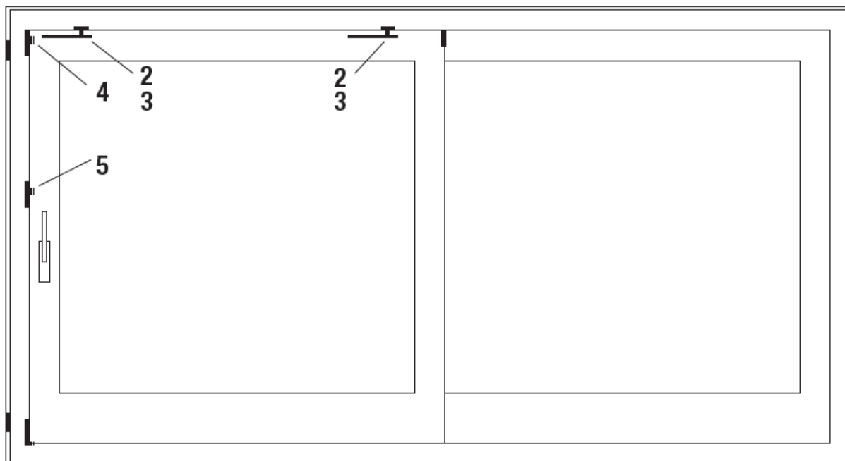
Bild: Hebe-Schiebe-Kipp-Tür
