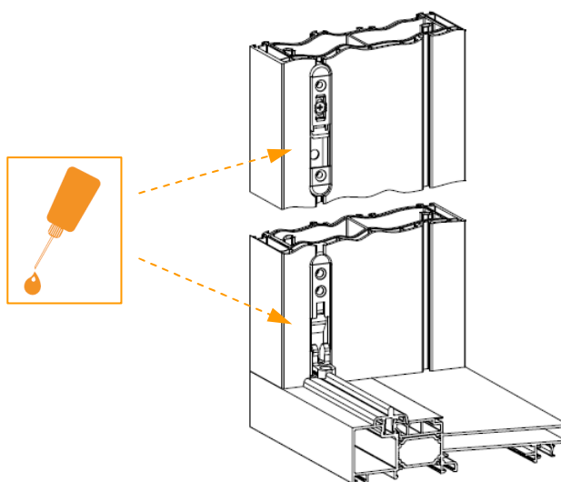
Hebe-Schiebe-Kipp-Tür
