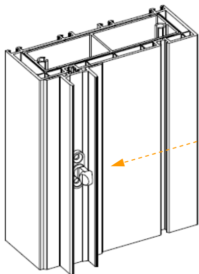
Hebe-Schiebe-Tür
